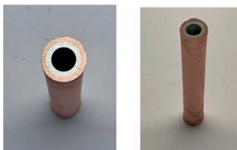
Figura 88. Amostra de alumínio após crescimento do filme de cobre.
