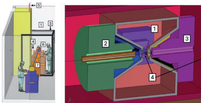
Figura 61 - (Esquerda) Vista da estação experimental da SIBIPIRUNA. 1 – Estação Experimental destinada a experimentos com amostras NB4, 3 – ‘bio-bolha’ de proteção de isolamento da estação experimental BSL4, 4 – tubo para transferência de amostras, 5 – tubos de alimentação do sistema de esterilização, 6 – Estação Experimental, 7 – Detector. (Direita) Design conceitual da Estação Experimental de Amostras. 1 - Módulo de Posicionamento da Amostra, 2 - Subsistema Óptico para focalização, 3 - Subsistema Óptico para demagnificação, 4 - Módulo do Suporte de Amostras
