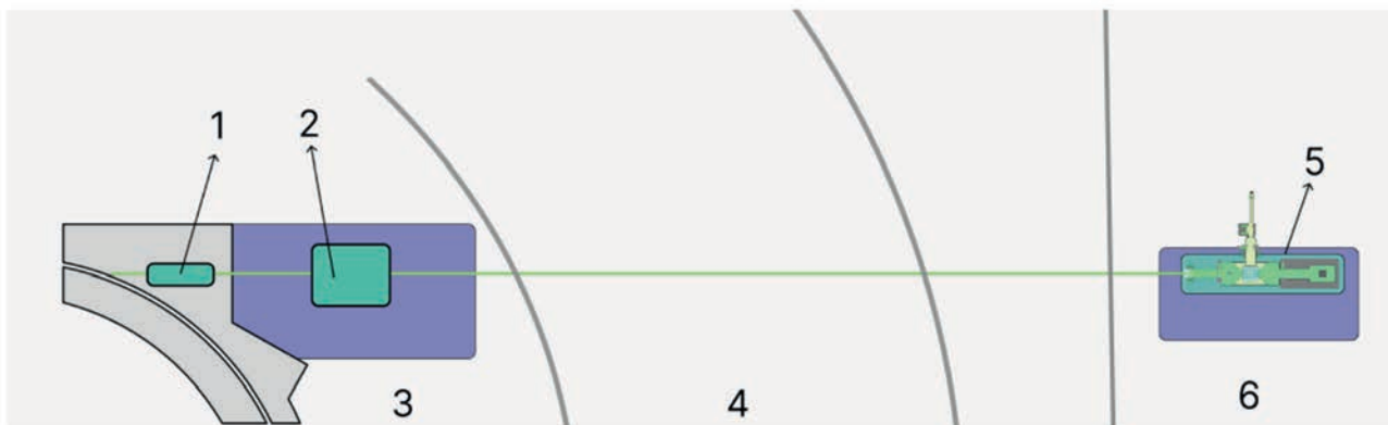
Figura 62 - Layout geral TIMBÓ e disposição dos prédios do Sirius e Orion. (1) Ondulador; (2) monocromador (DCM) dentro da cabana óptica; (3) piso de alta estabilidade do Sirius; (4) Hall experimental do Sirius; (5) estação experimental em nível de biossegurança 4; (6) prédio do Orion.
