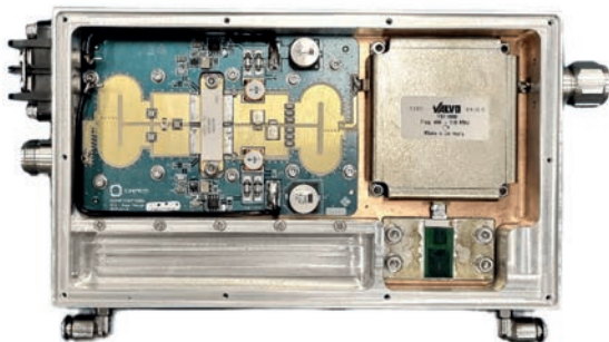
Figura 102: Amplificador de estado sólido com transistor BLF978P projetado no LNLs.
