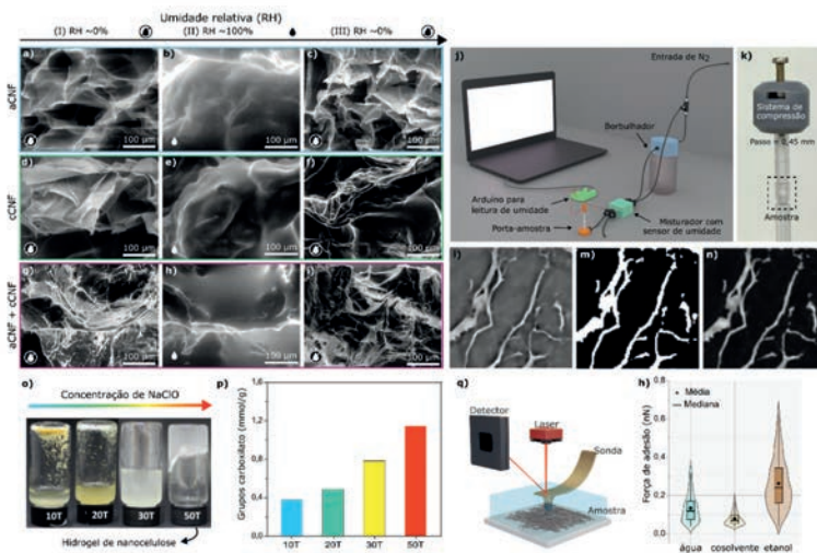
Figura 34 - Imagens de ESEM de criogéis preparados com (a) aCNF; (b) aCNF + cCNF; (c) cCNF. Os criogéis foram analisados em RH de 10, 100 e 10% (após condensação de água). Análise de \mu CT in situ com controle de umidade e deformação: (j) montagem experimental; (k) porta-amostra para compressão de criogéis; (l-n) treinamento de uma rede neural para segmentação de imagens: (l) área de interesse, (m) label de referência, (n) mapa de probabilidade gerado no treinamento. Produção de aCNFs a partir do bagaço de cana-de-açúcar em única etapa com NaClO 10, 20, 30 e 50 mmol/g de biomassa: (o) amostras após tratamento; (p) concentração de grupos carboxilatos determinados por titulação condutimétrica; (q) ilustração esquemática do sistema experimental utilizado para as medidas de espectroscopia de força e (b) gráficos de violino e boxplot para a força de adesão obtidos a partir de 1024 curvas de força-distância.
