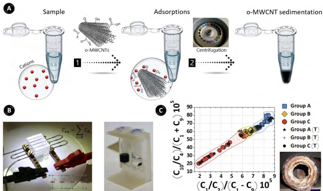
Figura 102. Sensor não seletivo e machine learning para análises em meio ambiente. Esquema do método para interação entre íons e nanotubos (A), sensor para análise do sobrenadante após sedimentação dos nanotubos, à esquerda, e frasco com nanotubos dispersos e sedimentados, à direita, (B) e dado obtido por machine learning referente à discriminação de dezenas de amostras de águas com metais em concentrações abaixo (grupo A) e acima (grupos B e C) dos limites aceitos pela OMS (C).
