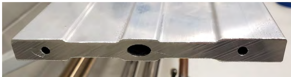
Figura 152. Perfil de alumínio extrudado na liga 6063-T6 para a fabricação das câmaras do Delta 52.
