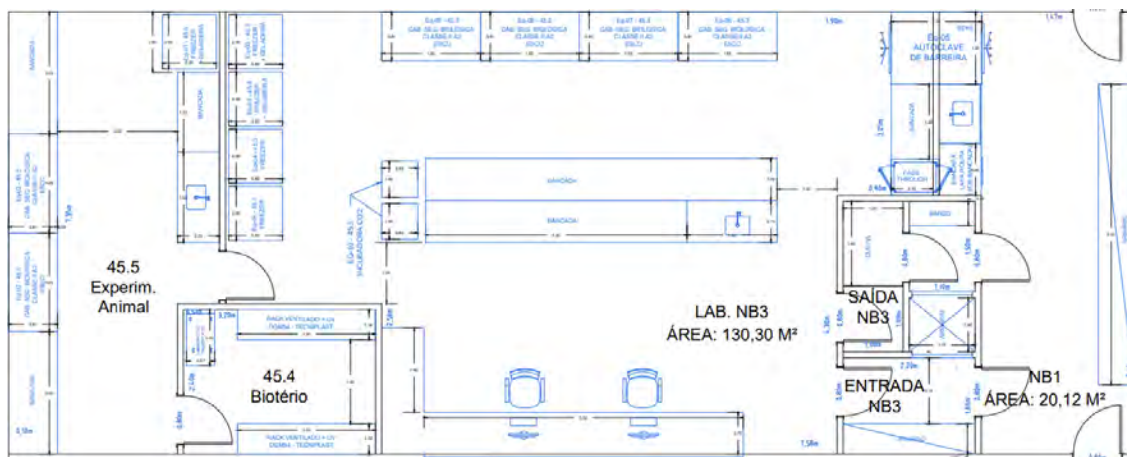
Figura 207. Proposta conceitual de ocupação do laboratório NB3.
