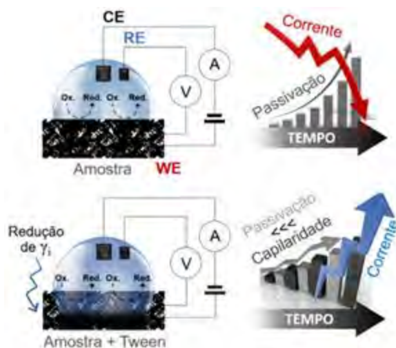
Figura 135. Com o avanço gradual da amostra nos poros do eletrodo, a amplificação da corrente se dá numa magnitude superior ao efeito da passivação pelas proteínas presentes nas amostras.
