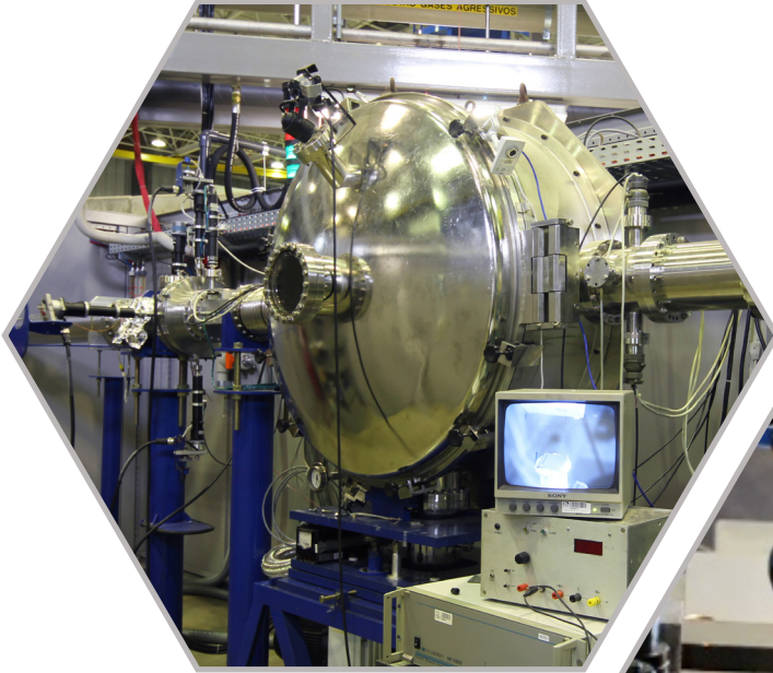
Instrumentação científica da linha de luz XRD1
