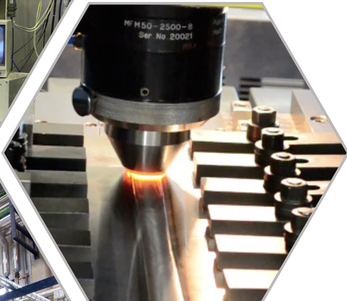
Soldagem por Atrito com Pino Não-consumível
